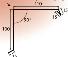
Oberer Windträger / Ortgang
